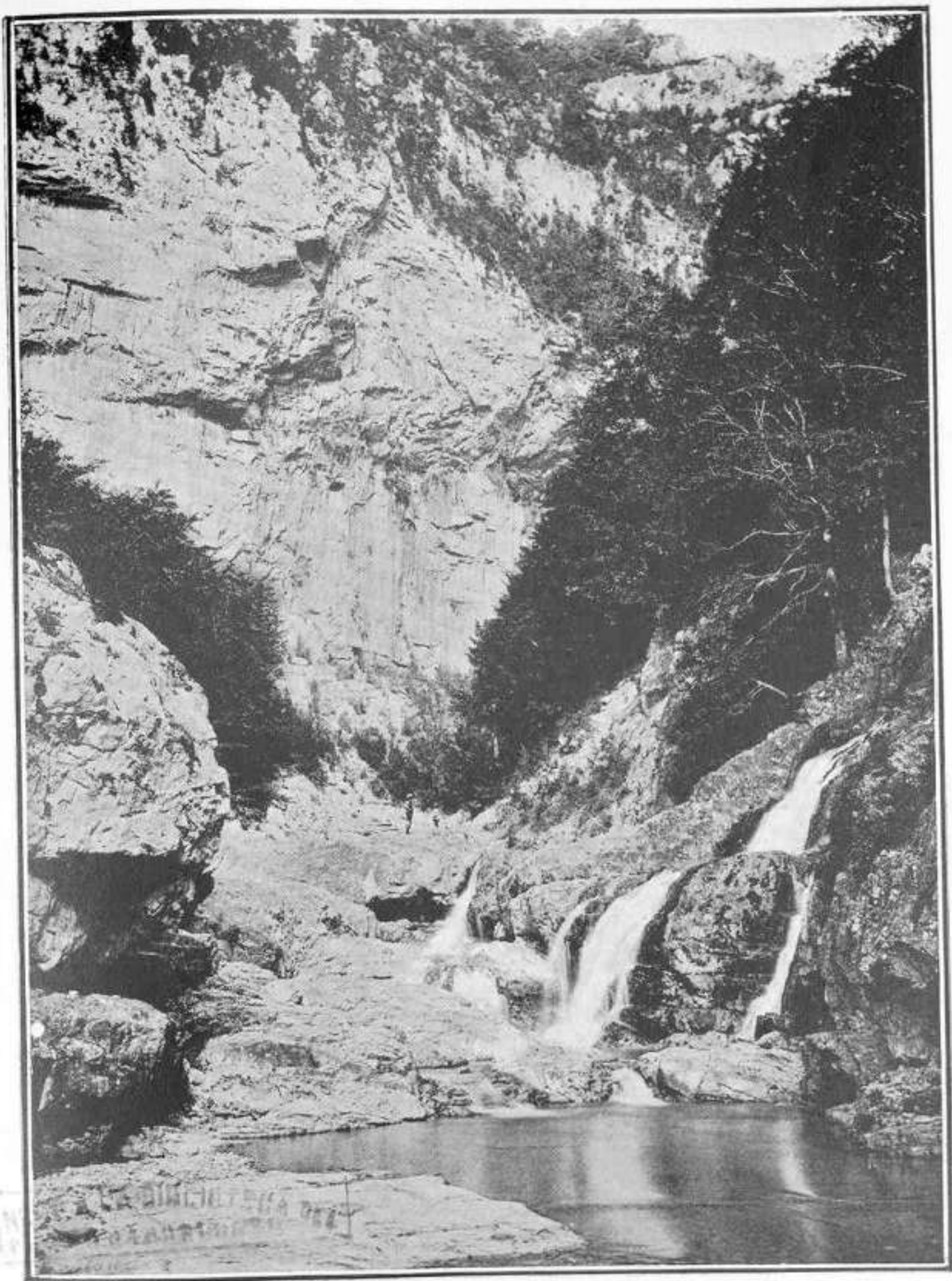
Interior de la garganta de Escoain. — La fuente origen del río Yaga.
